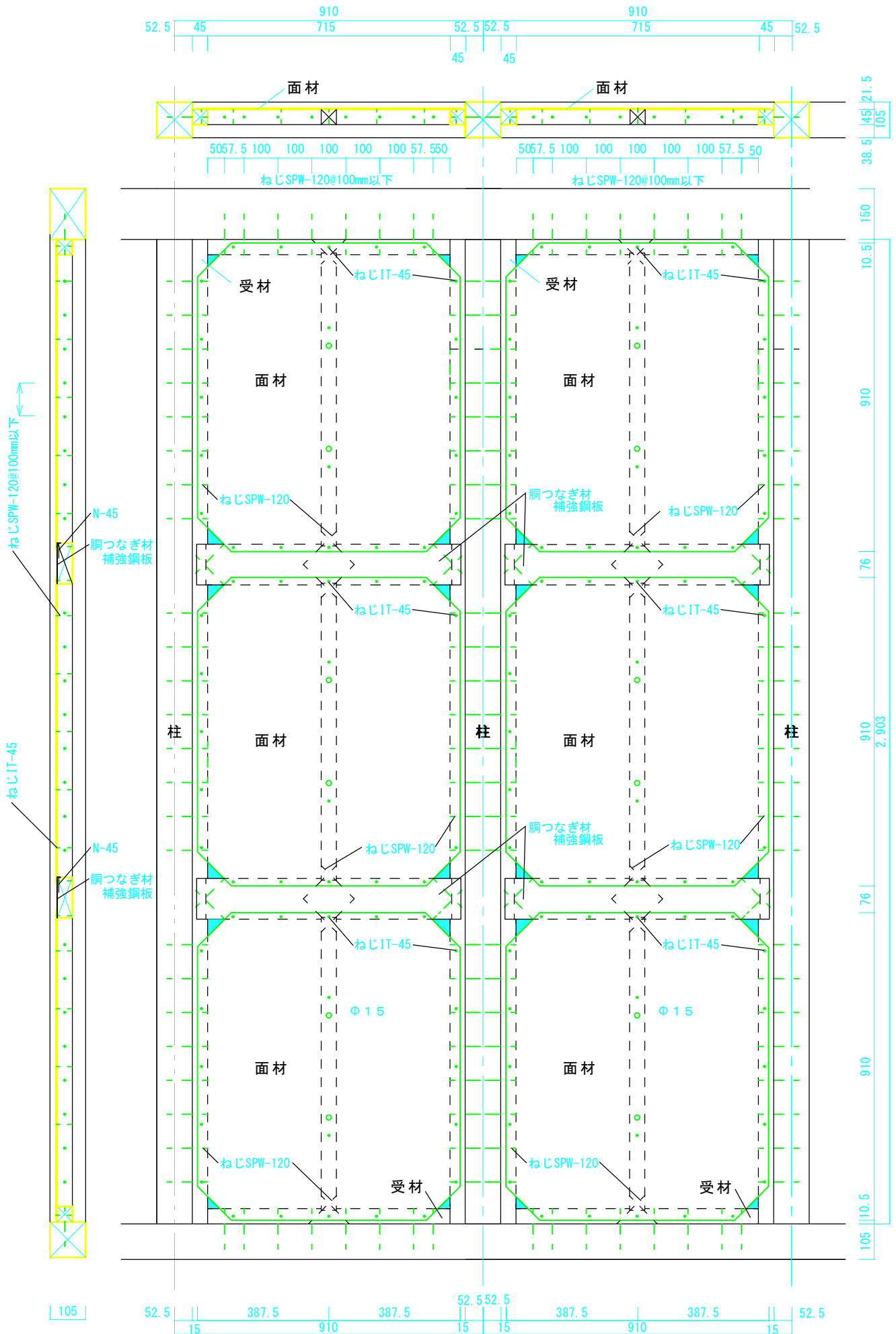
【図3】連続使用施工詳細図（面材間すき間最大）
