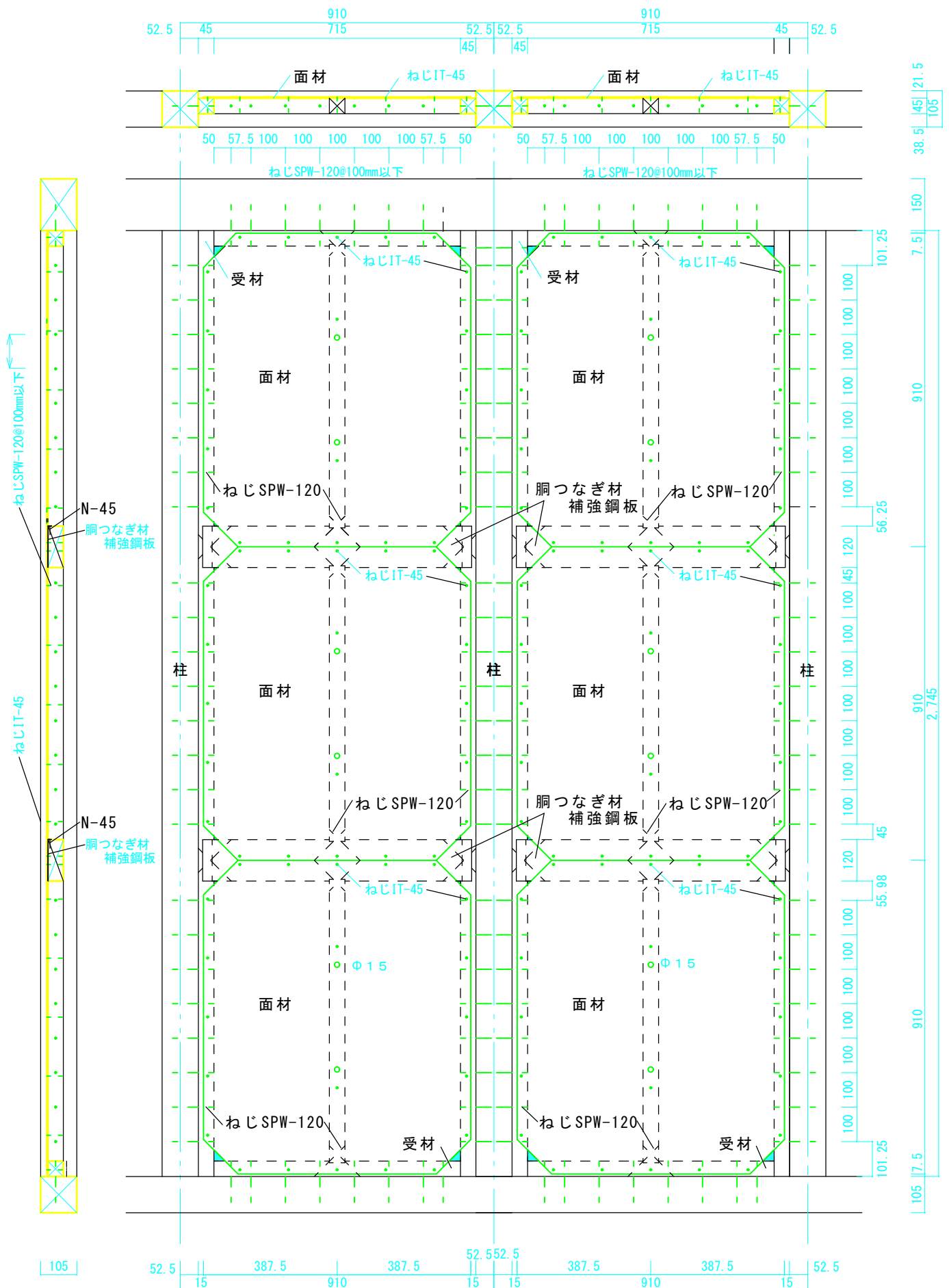
【図 4】連続使用標準施工図（面材間すき間なし）
